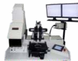
Полуавтоматическая установка совмещения и экспонирования фоторезиста
