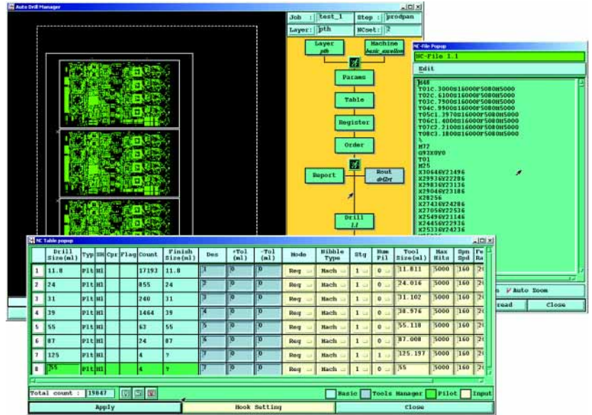
Рисунок 13 Подготовка файлов сверления с помощью модуля
