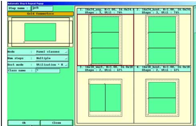
Рисунок 6 Выбор шаблона мультиплицирования топологии
