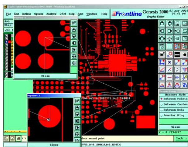
Рисунок 3 Измерение расстояния между двумя объектами с использованием вспомогательных увеличительных окон
