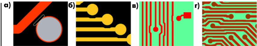
Рисунок 10 Результат применения различных автоматизированных процедур по устранению нарушений зазоров
