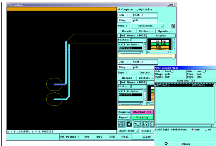
Рисунок 12 Сравнение двух списков соединений (исходного и конечного) позволило выявить замыкание между двумя проводниками
