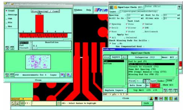
Рисунок 9 Оценка статистического распределения значений нарушений зазоров на сигнальных слоях платы
