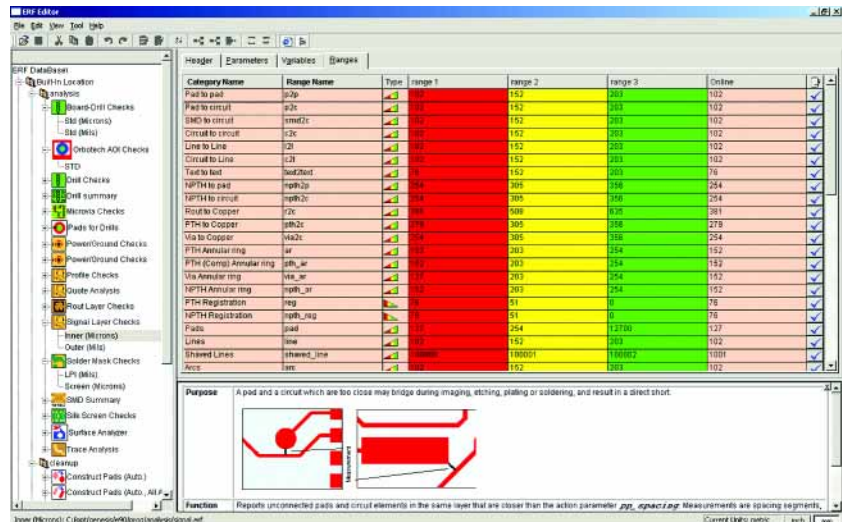
Рисунок 14 Новый модуль ERF Editor позволяет оперативно управлять наборами параметров различных процедур системы Genesis 2000 Auto Drill Manager
