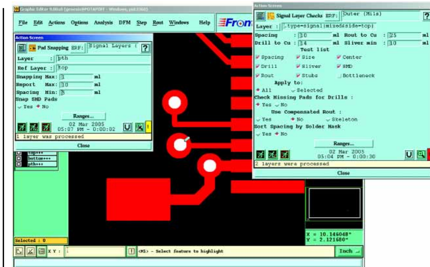
Рисунок 11 Проверка центровки отверстий сверления относительно центров контактных площадок
