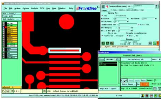
Рисунок 8 Автоматическое преобразование неправильно нарисованных контактных площадок во флэши
